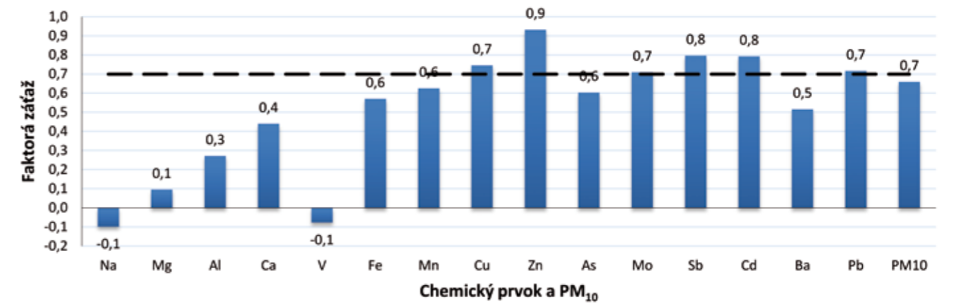
Faktorová záťaž premenných (chemického prvku) k faktoru 1 – lokálne spaľovanie a nevýfukové emisie (obrus pneumatík) v roku 2013 pri diaľnici D1 Predmier
