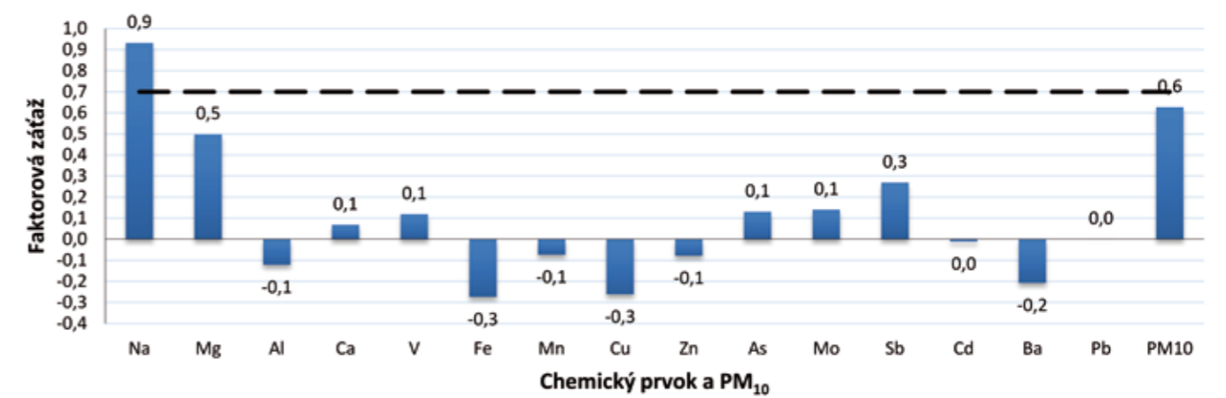
Faktorová záťaž premenných (chemického prvku) k faktoru 3 – cestný prach a materiál zimného posypu v roku 2013 pri diaľnici D1 Predmier
