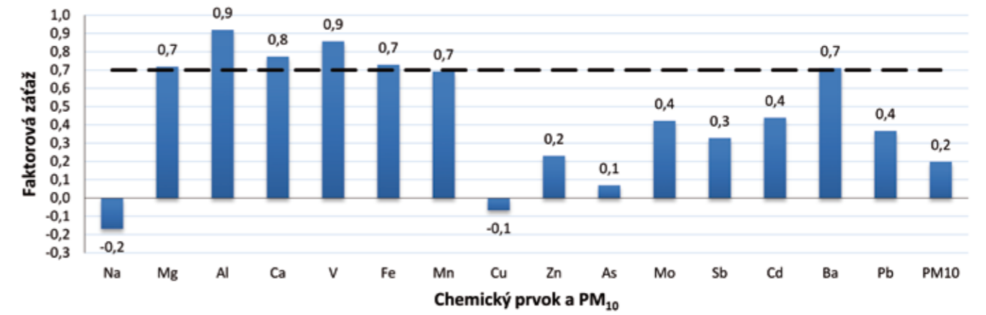
Faktorová záťaž premenných (chemického prvku) k faktoru 2 – výfukové emisie (nafta, mazacie oleje) a zemská kôra v roku 2013 pri diaľnici D1 Predmier
